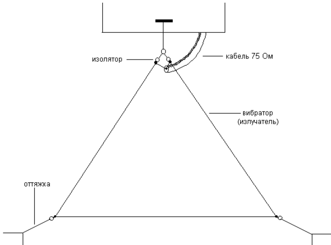
Рис.2.12. Антенна «треугольник»
