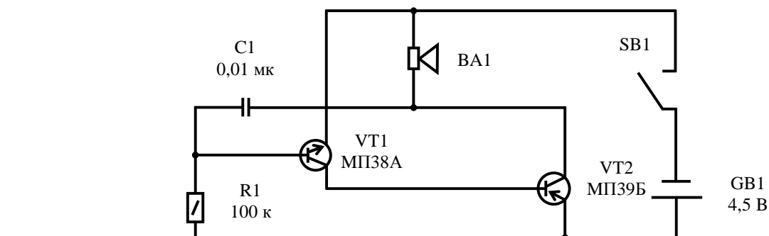
Рис.8.4. Схема звукового генератора
